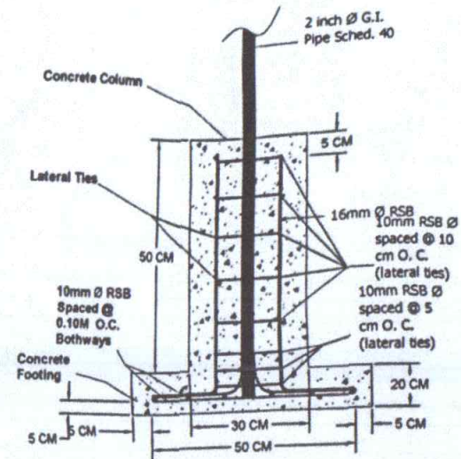
SECTION "1E" SCALE: NTS
